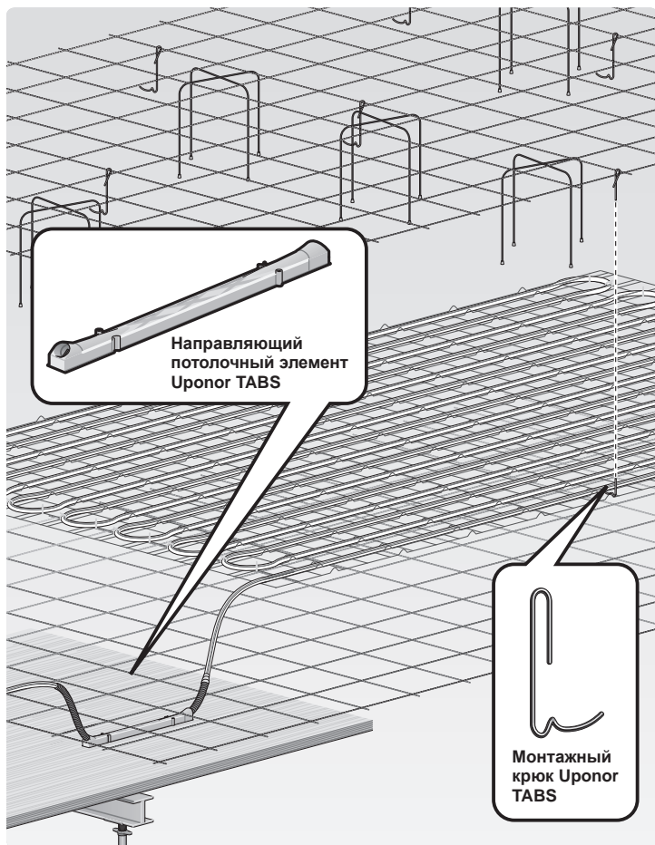
Послойный вид изготавливаемого на стройплощадке железобетонного перекрытия с системой Upronor TABS Contec
