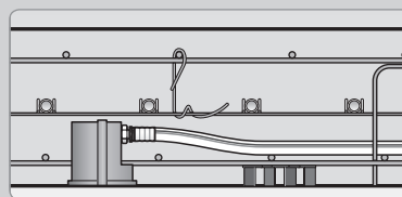
Терморозетка Upronor Contec TS
